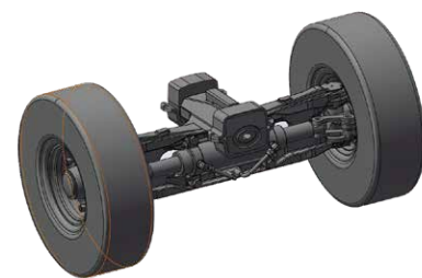
Gusseiserne Lenkachse
